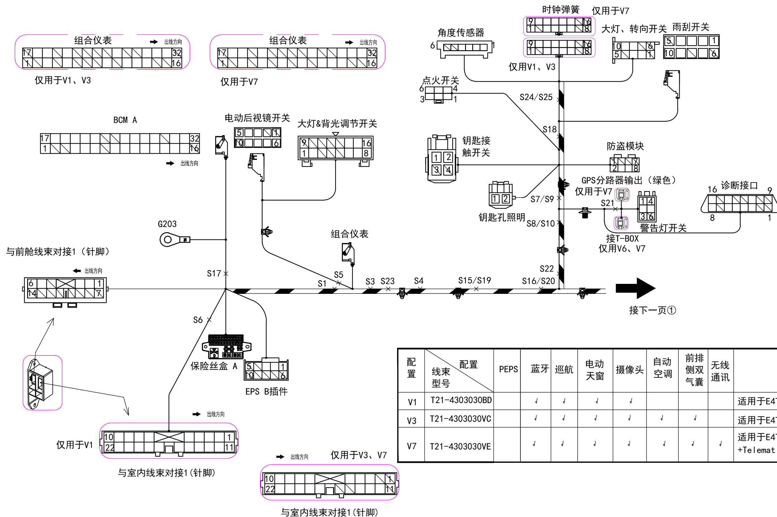
2.11、仪表线束插件端子图一
